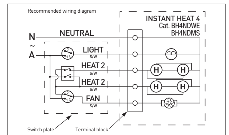
Fig 8. Wiring diagram
